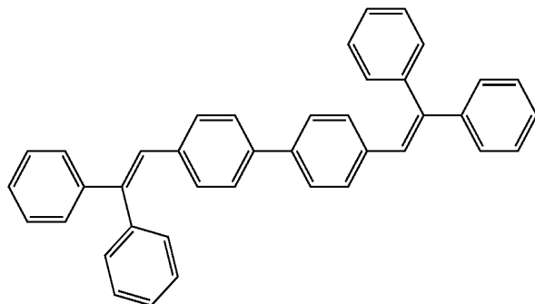
DPVBi
