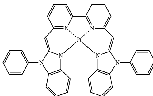
PD2
