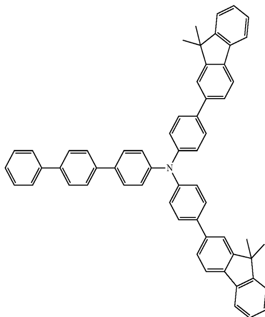
HT20
